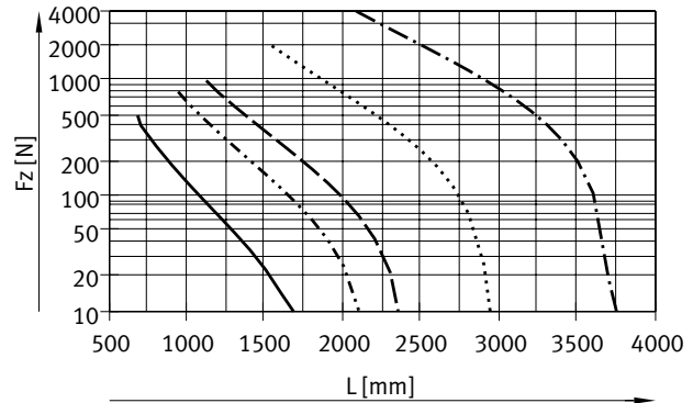
Kraft F_z
